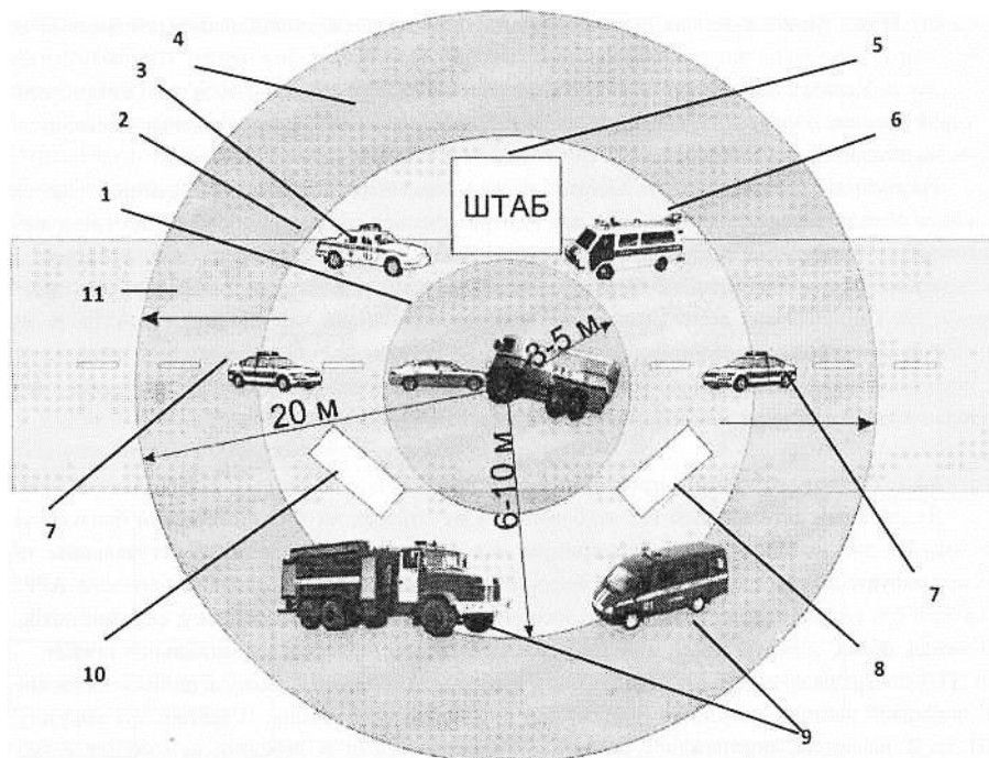
Рис. 3.3 - Типова схема організації місця проведення рятувальних робіт:
